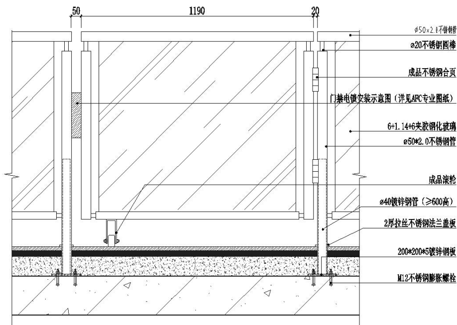
① 边门立面图 1:10
