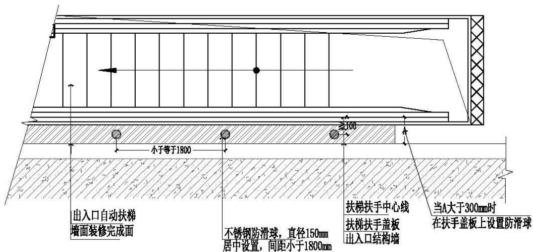
出入口靠墙扶梯扶手盖板防滑球设置要求
