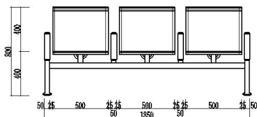
站台层座椅正立面图 1:20
