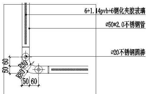
③ 转角大样图 1:10
