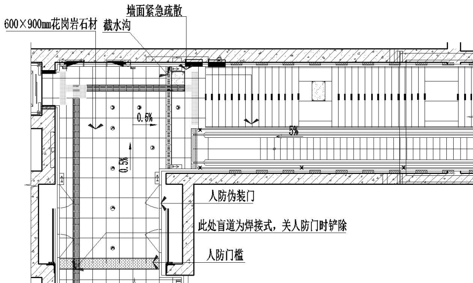
人防段平面示意图 1:100
