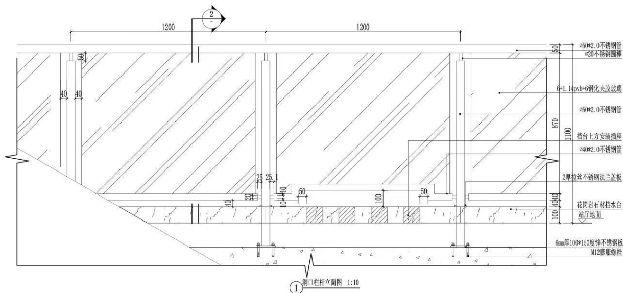
附图 2: 洞口防护栏杆大样图
