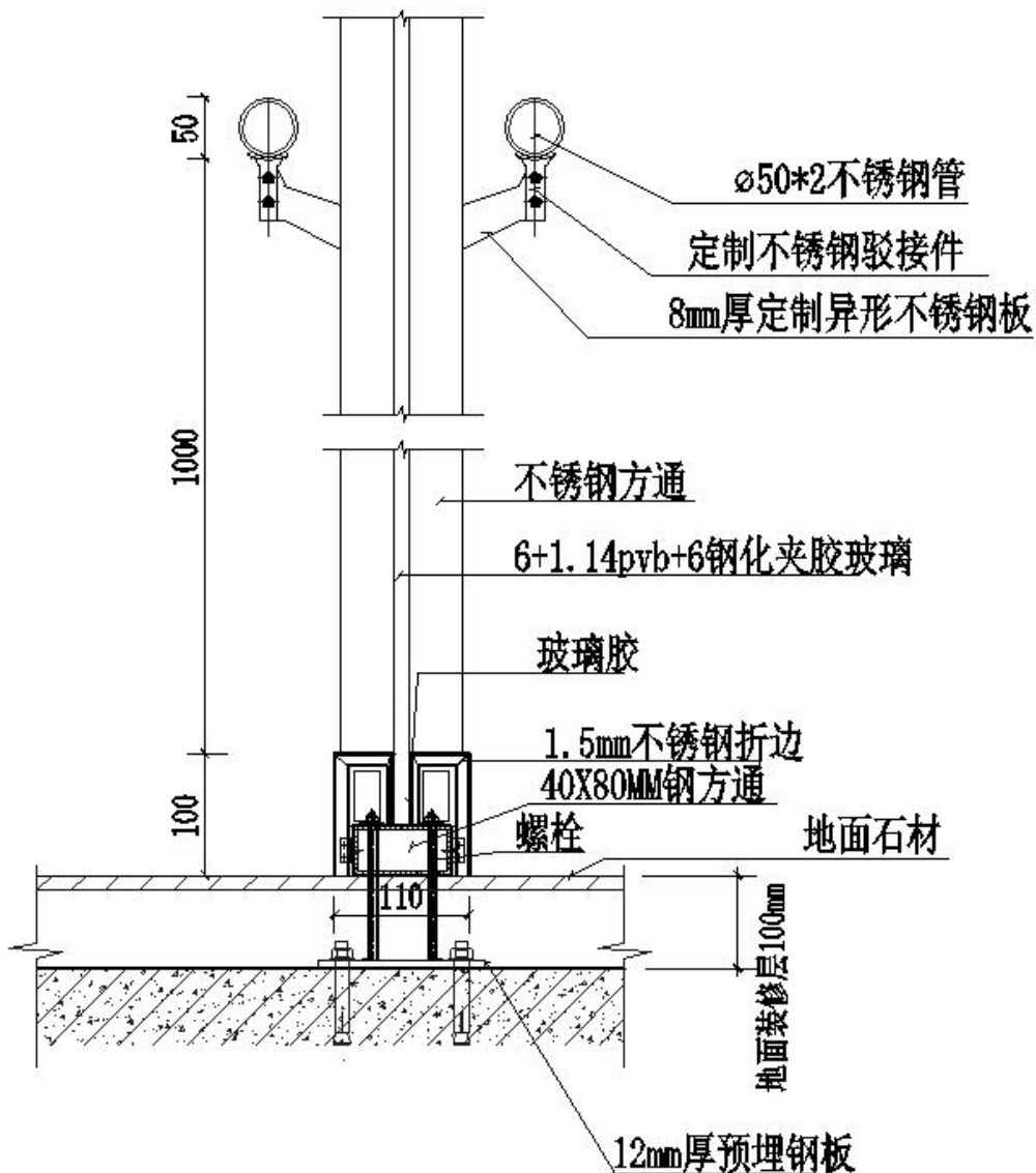
1-1剖面图 1:10
