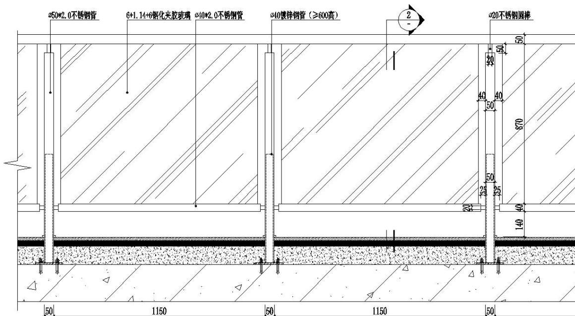
① 分区栏杆立面图 1:10
