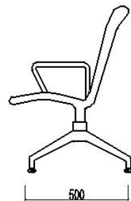
站台层座椅侧立面图 1:20
