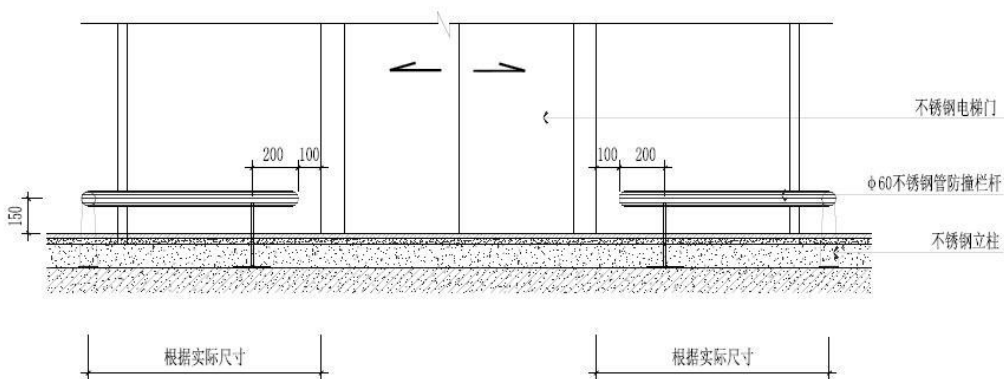
无障碍垂直电梯防撞栏杆正立面图 1:20
