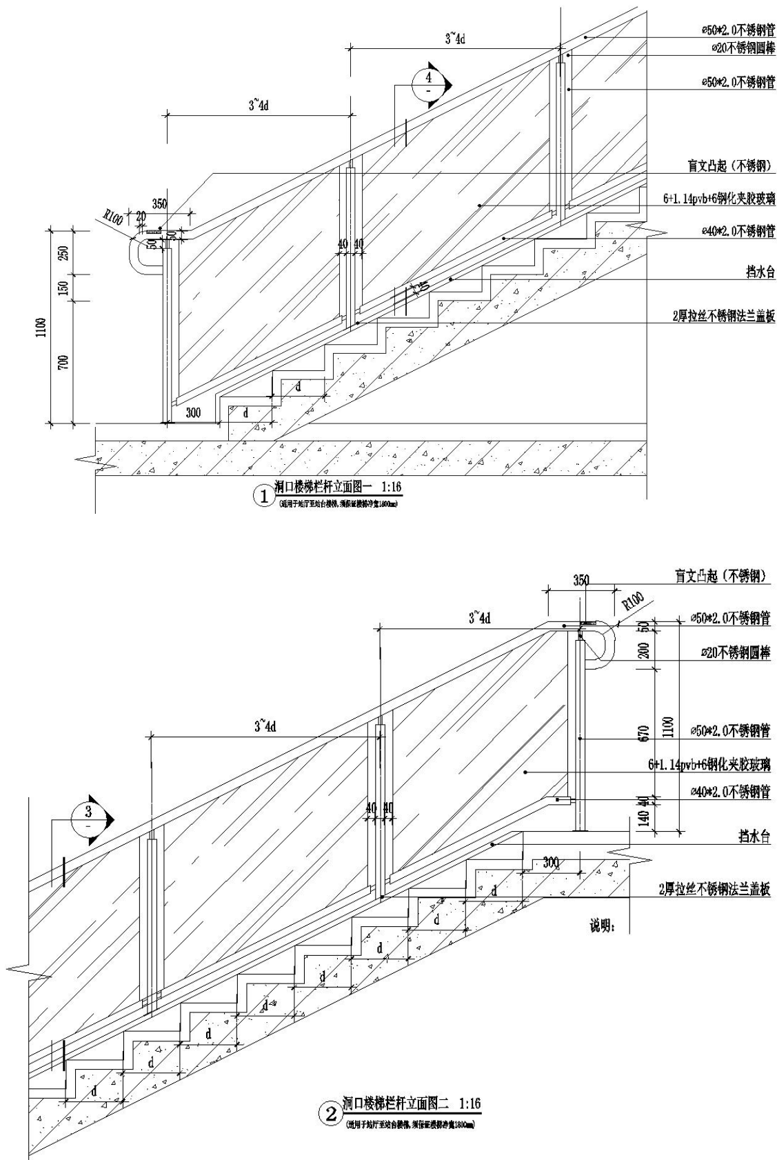
附图 3：楼梯栏杆大样图
