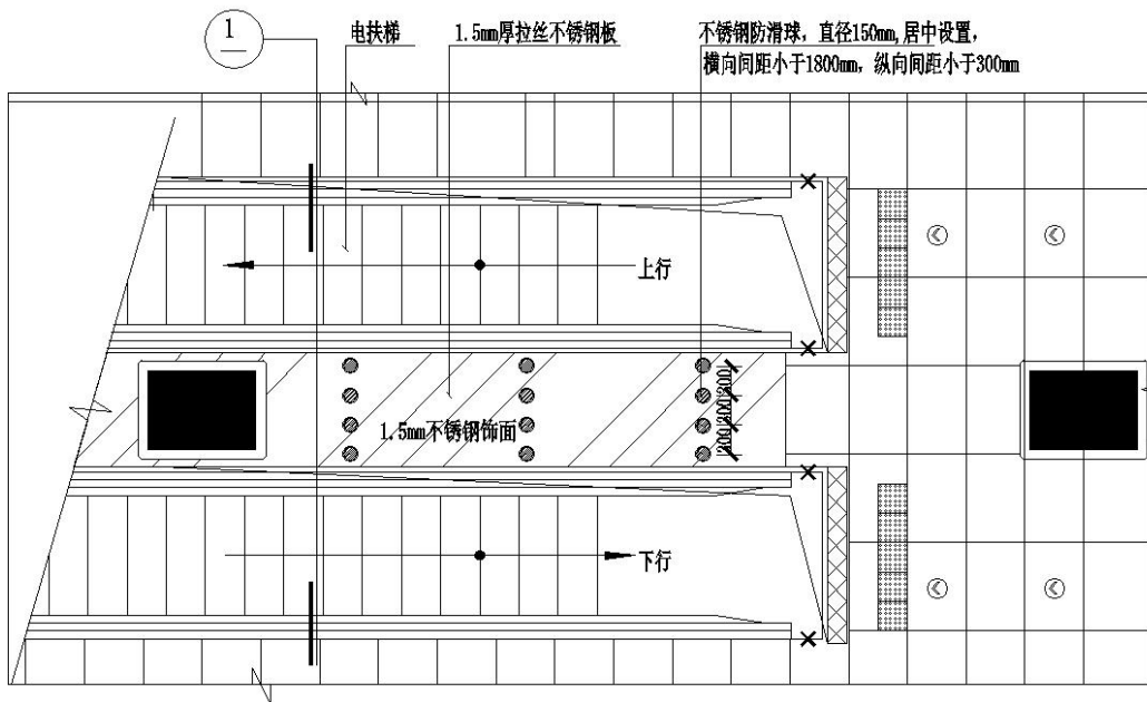
站厅下站台双扶梯防滑球设置要求
