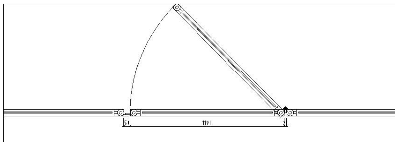
① 边门平面图 1:10
