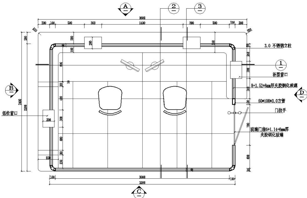
客服务中心平面图 1:20
