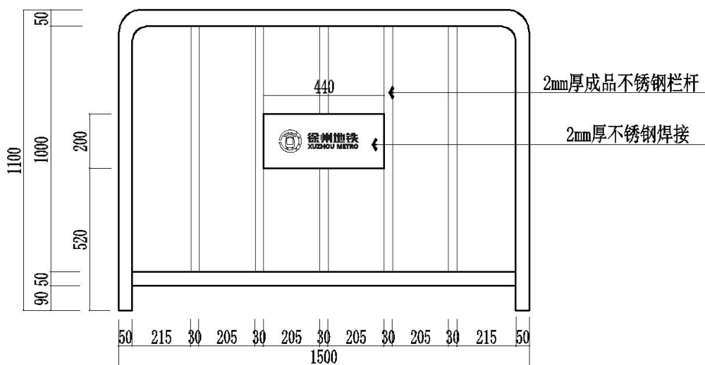
可移动栏杆正立面图 1:15
