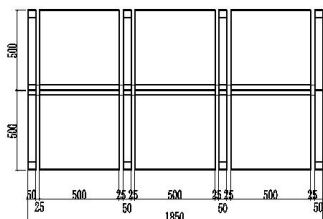
站台层座椅平面图 1:20
