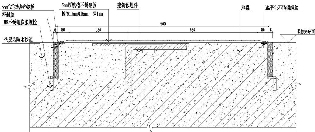
不锈钢人防门门槛剖面大样图 1:5
