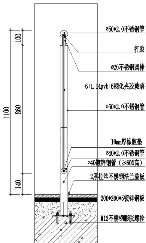
② 分区栏杆纵剖面图 1:10
