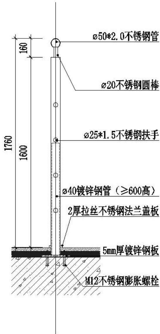
3 分流栏杆纵剖图 1:10
