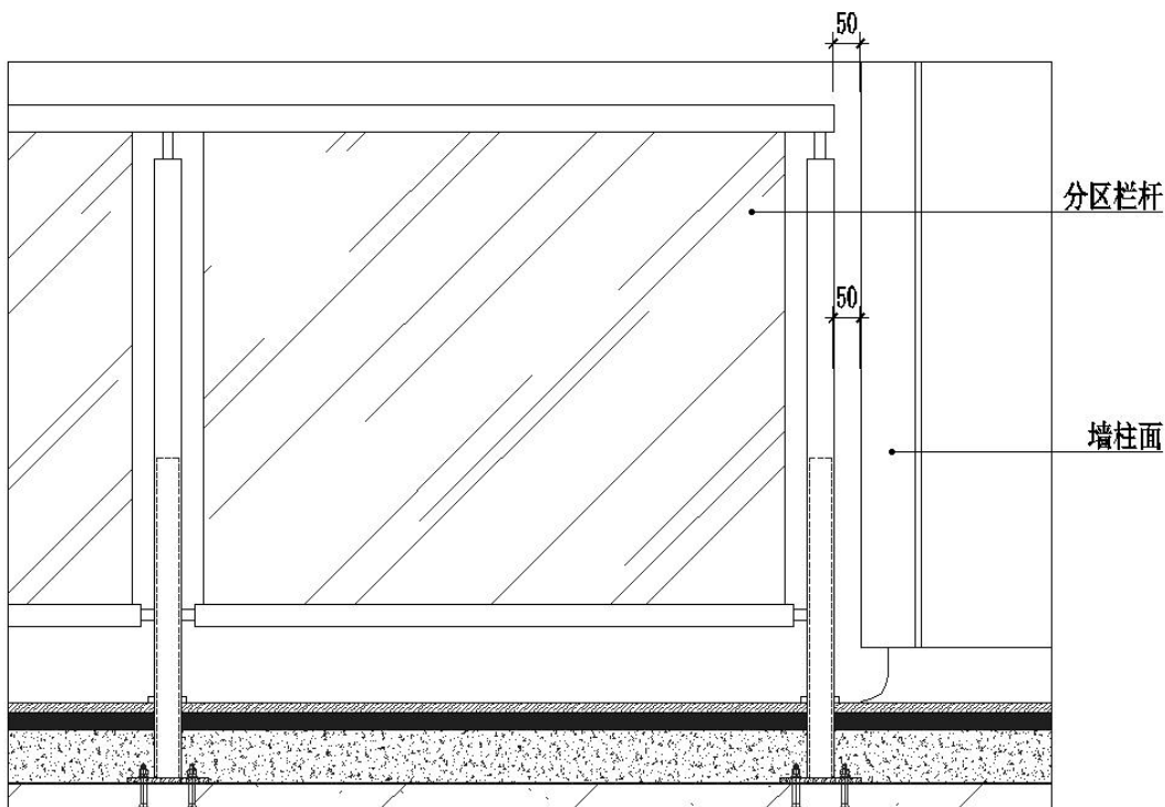
① 分区栏杆与墙柱面接口示意图 1:10
