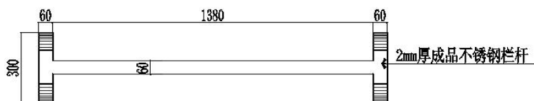
可移动栏杆平面图 1:15
