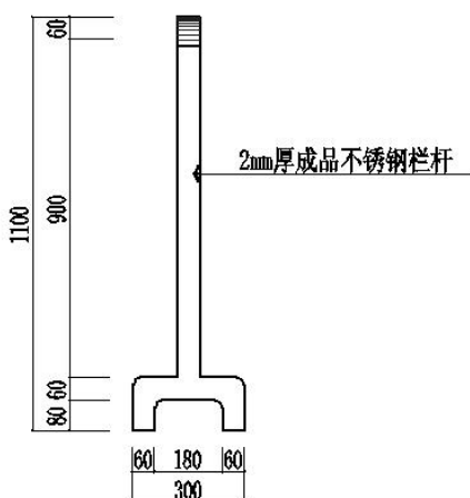
可移动栏杆侧面图 1:15
