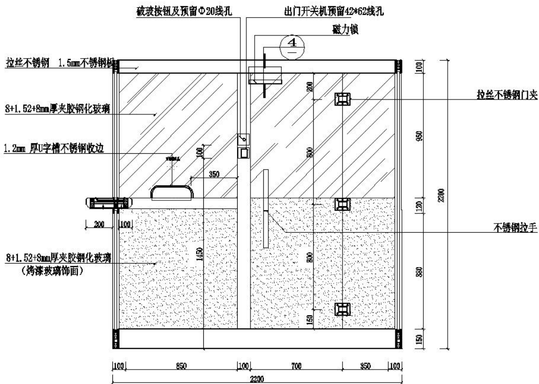
③ 客服中心-3剖面图 1:20
