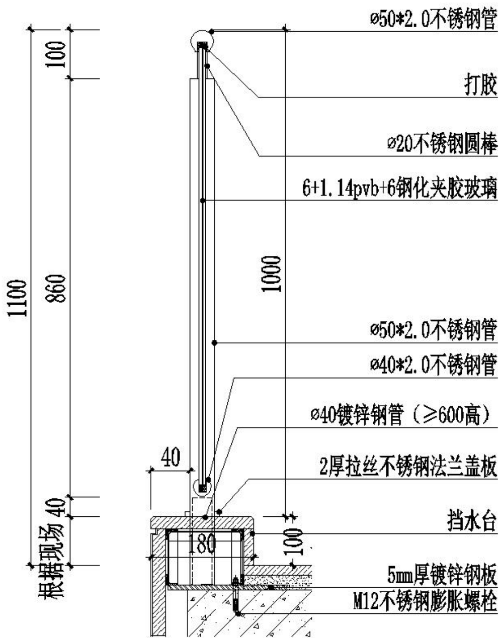
4 楼梯栏杆剖面图 1:10
