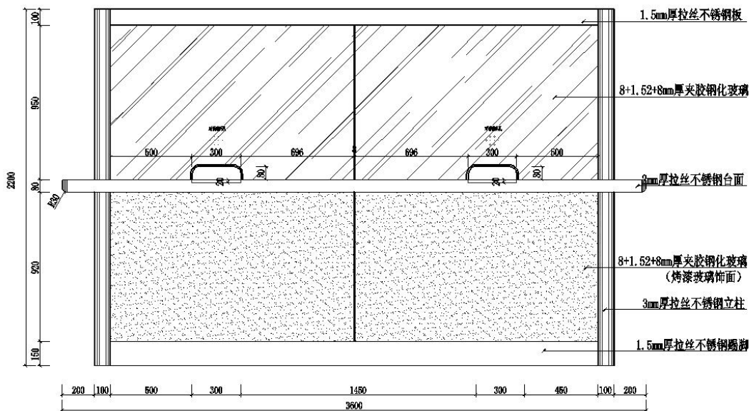
客服务中心 - A立面图 1:20
