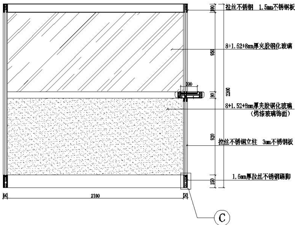
② 客服中心 -2剖面图 1:20
