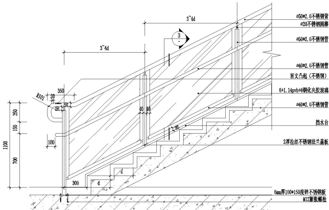
① 双扶手楼梯栏杆立面图一 1:16 (适用于出入口楼梯, 须保证楼梯净宽1800mm)
