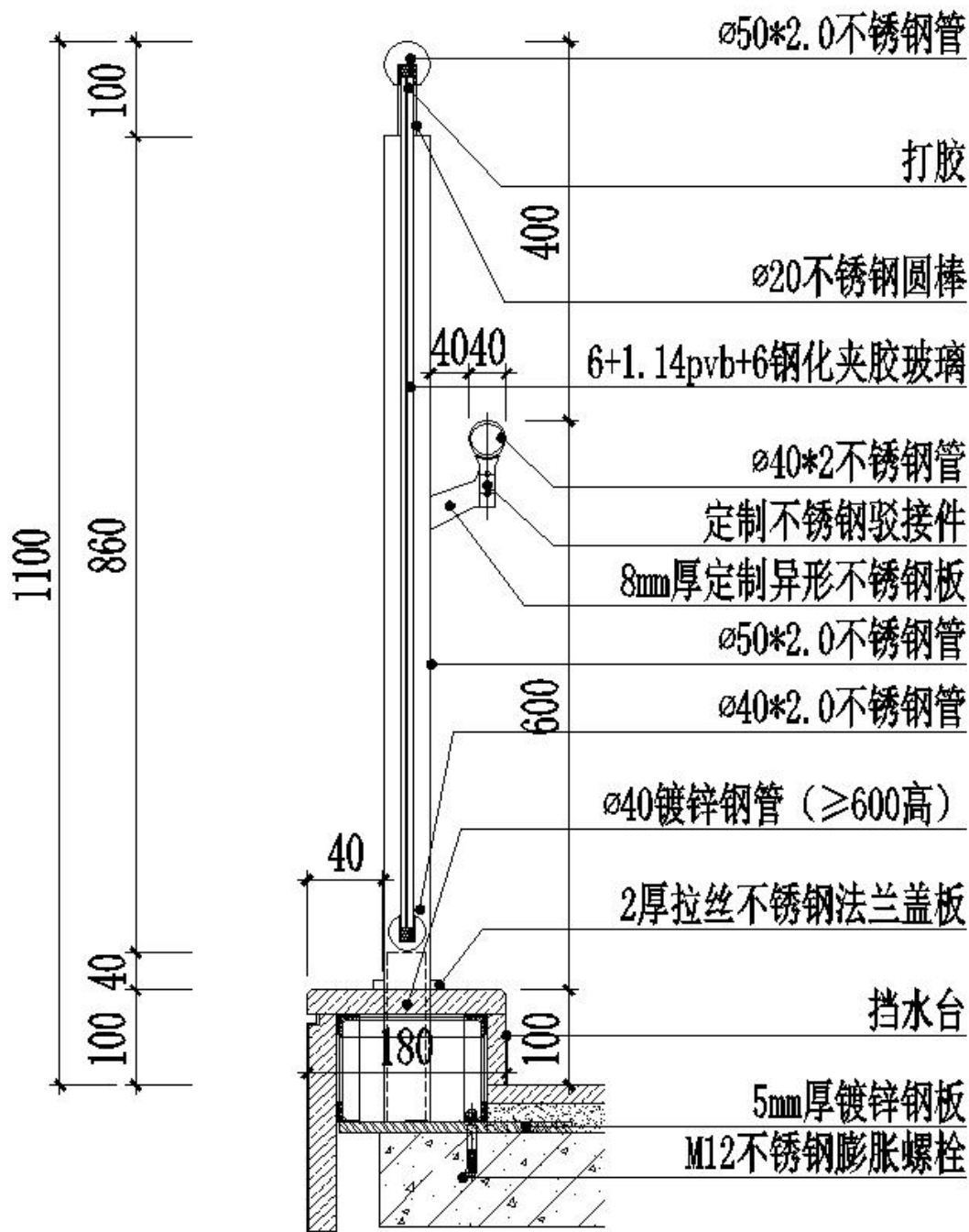
④ 双扶手楼梯栏杆剖面图 1:10
