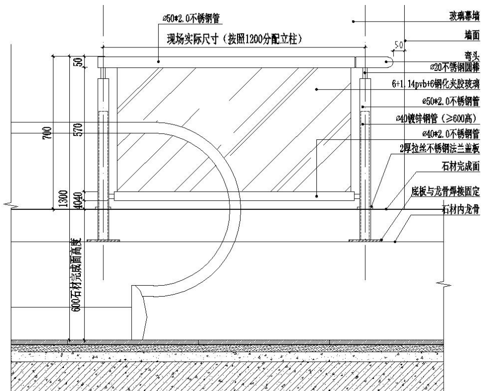
① 出入口栏杆正立面图 1:10
