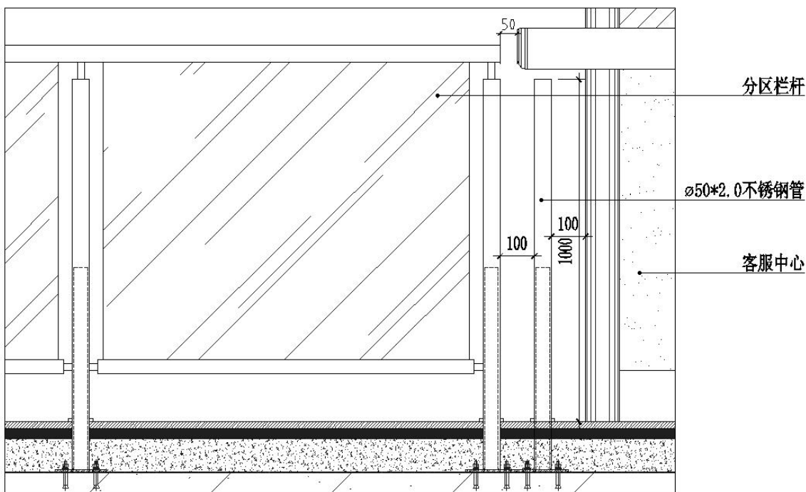
② 分区栏杆与客服中心接口示意图 1:10
