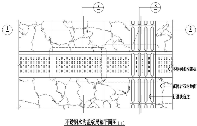
附图 15：不锈钢水沟盖板大样图
