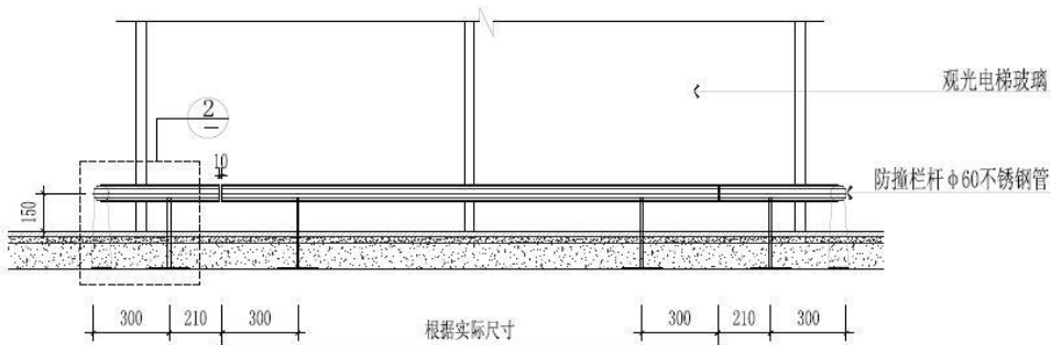
无障碍垂直电梯防撞栏杆侧立面图 1:20
