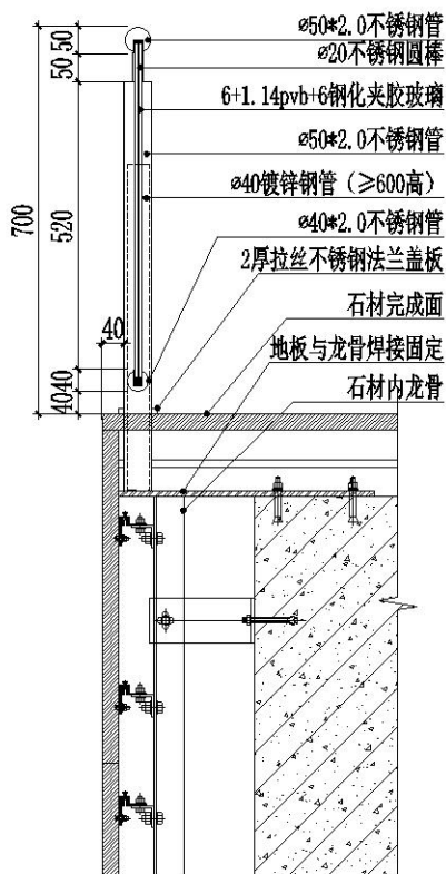
② 侧剖图 1:10
