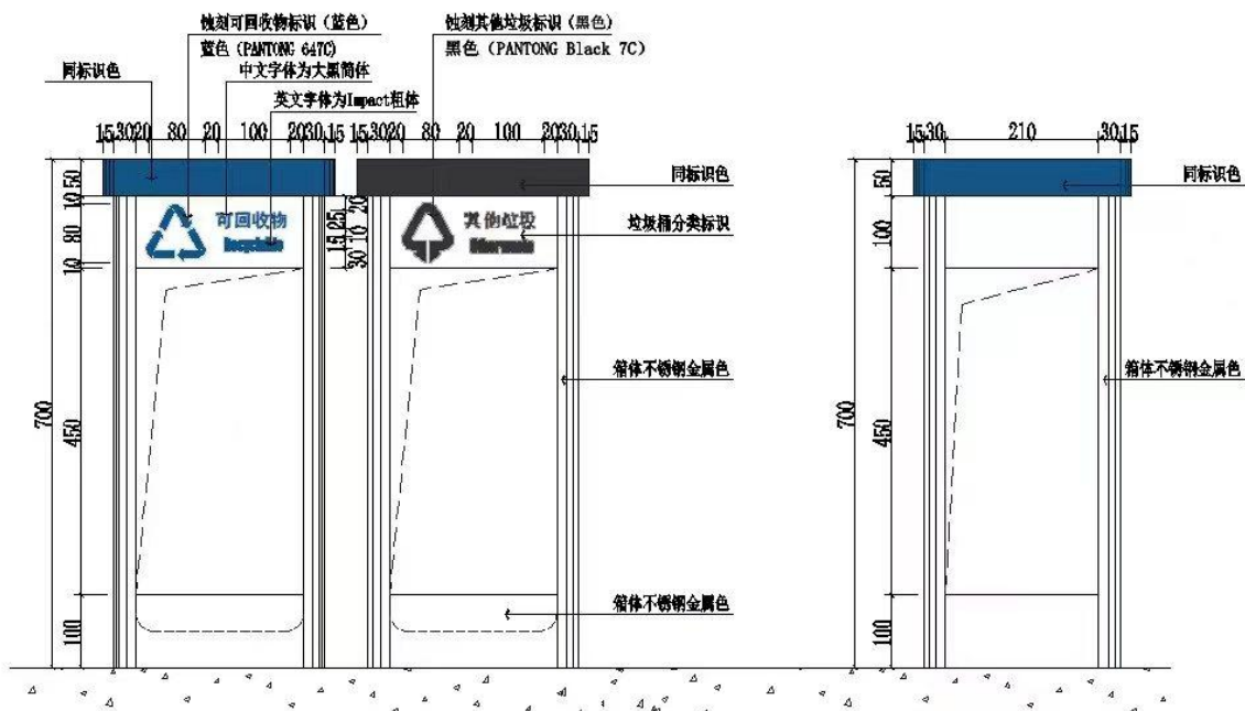
站厅、站台垃圾桶侧立面图 1:5
