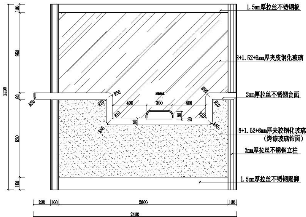
客服中心 - B立面图 1:20
