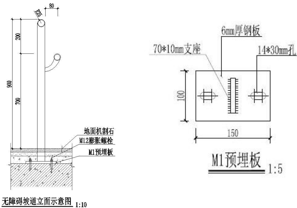
附图7：无障碍坡道栏杆大样图
