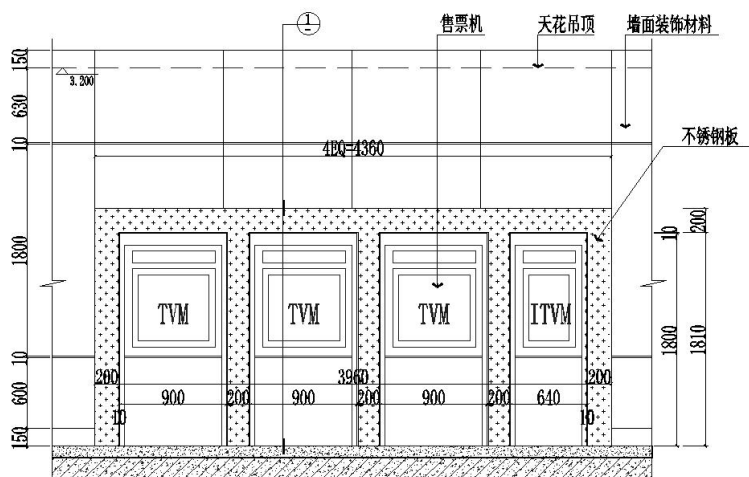
售票机立面图1:30
