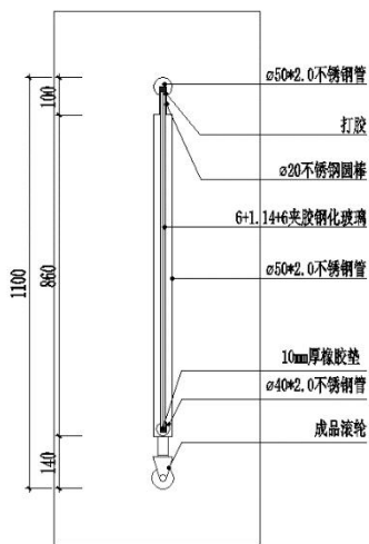
② 分区栏纵剖图 1:10
