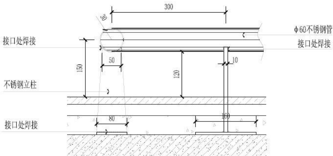
② 无障碍垂直电梯防撞栏杆局部大样图 1:5
