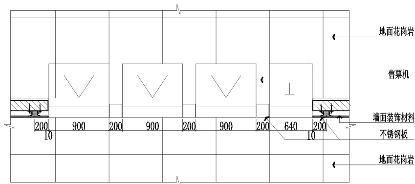
售票机平面图1:30
