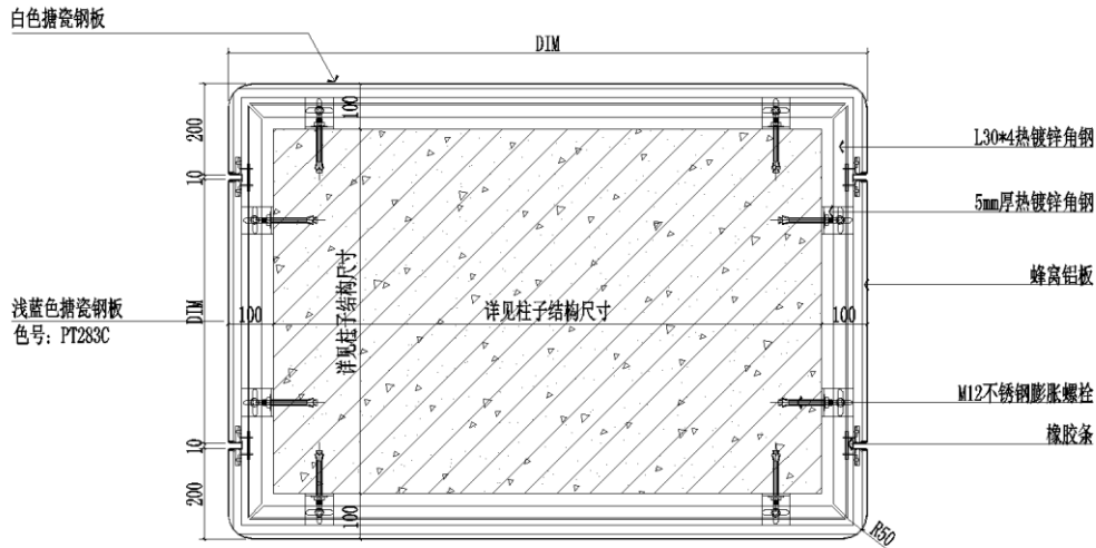
附图 2：标准柱面横剖面图
