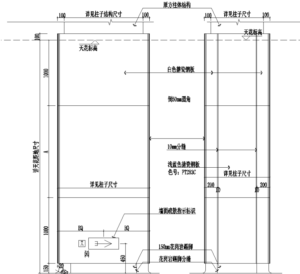
附图 1：标准方柱面立面图
