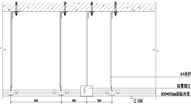
②卫生间铝扣板吊顶详图 1:10
