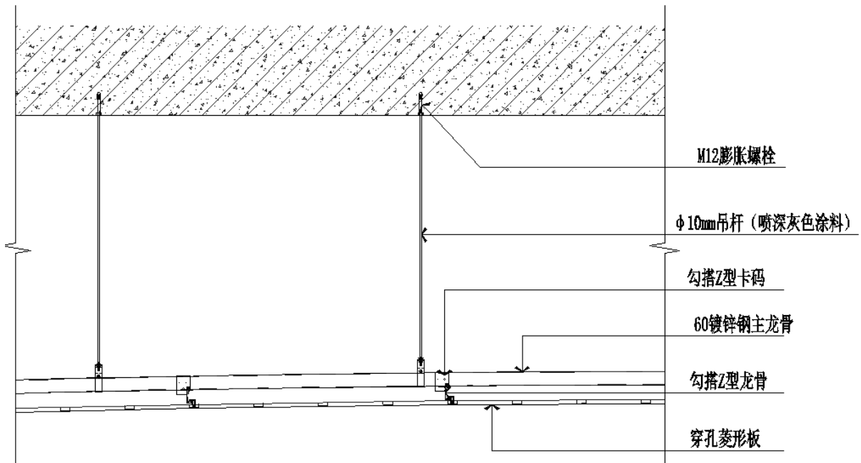
② 穿孔铝板天花纵向剖面图 1:10
