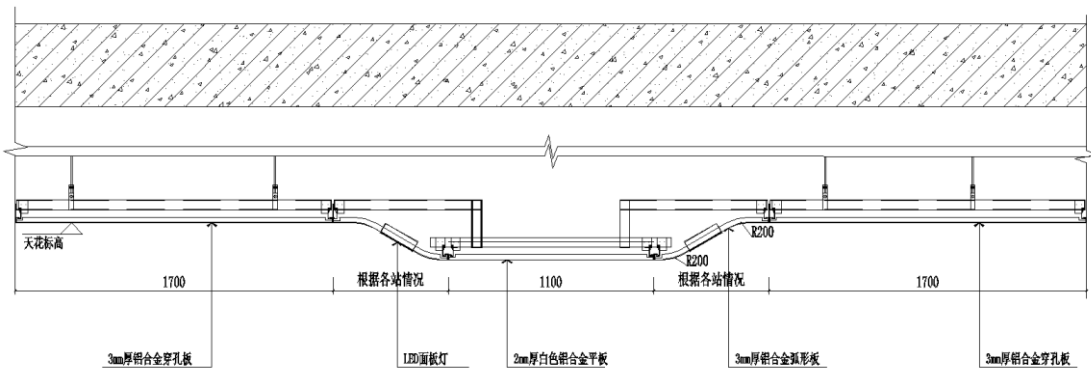
附图：标准站造型铝板吊顶大样图
