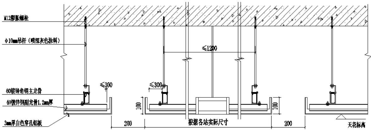
② 穿孔铝板天花纵向剖面图 1:10
