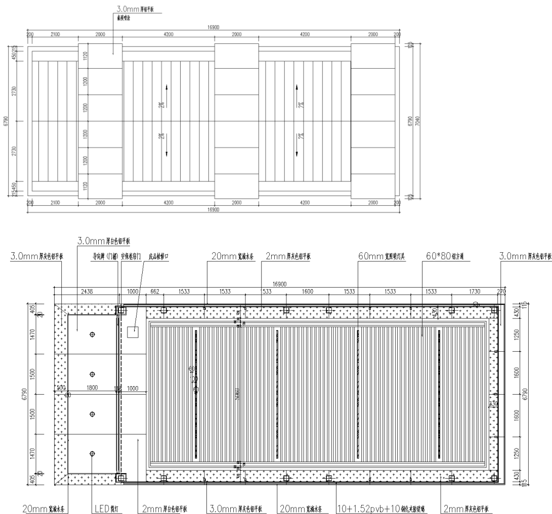
附图：出入口铝合金平板
